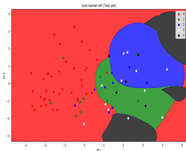
Fig-9.2 SVMRBF(Testset)
