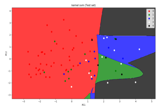
Fig-8.2 SVMPoly(Testset)
