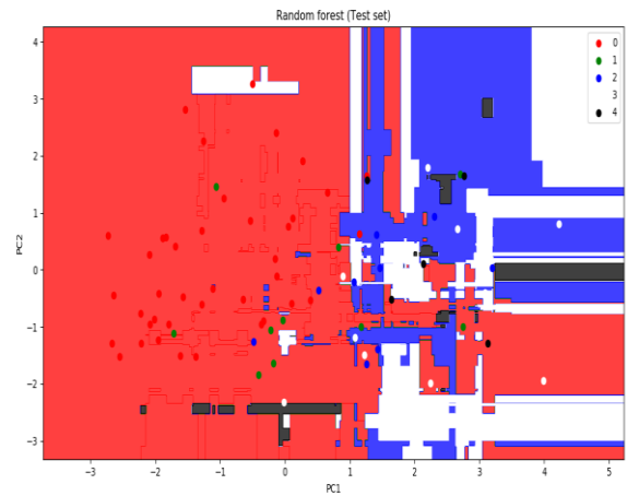
Fig-7.2 RandomForest(Testset)
