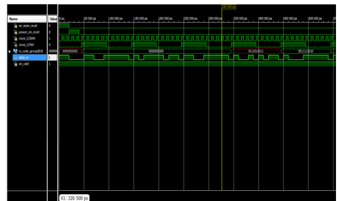
Figure9--SIPO.
